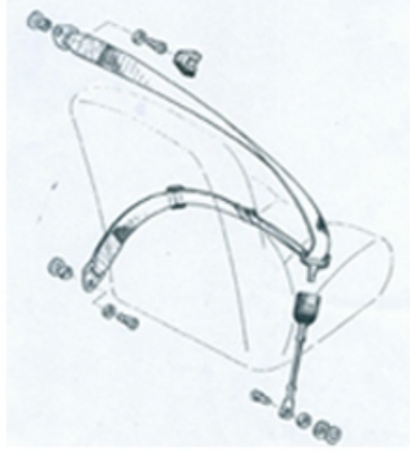
Pas bezpieczeństwa trzypunktowy statyczny typ A
